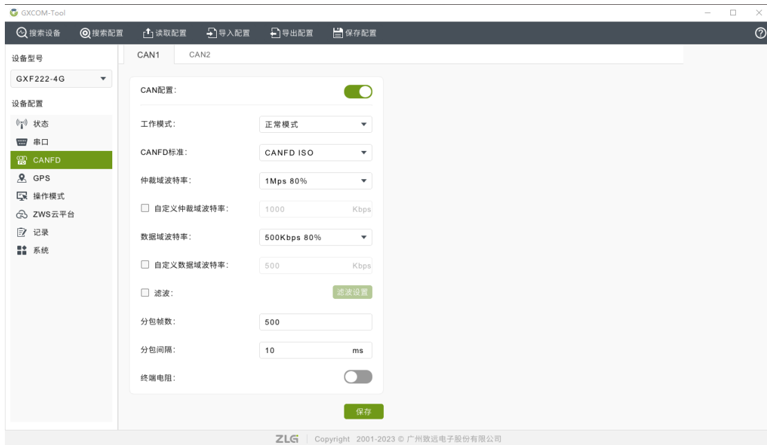
图 2.12 CAN FD 配置
