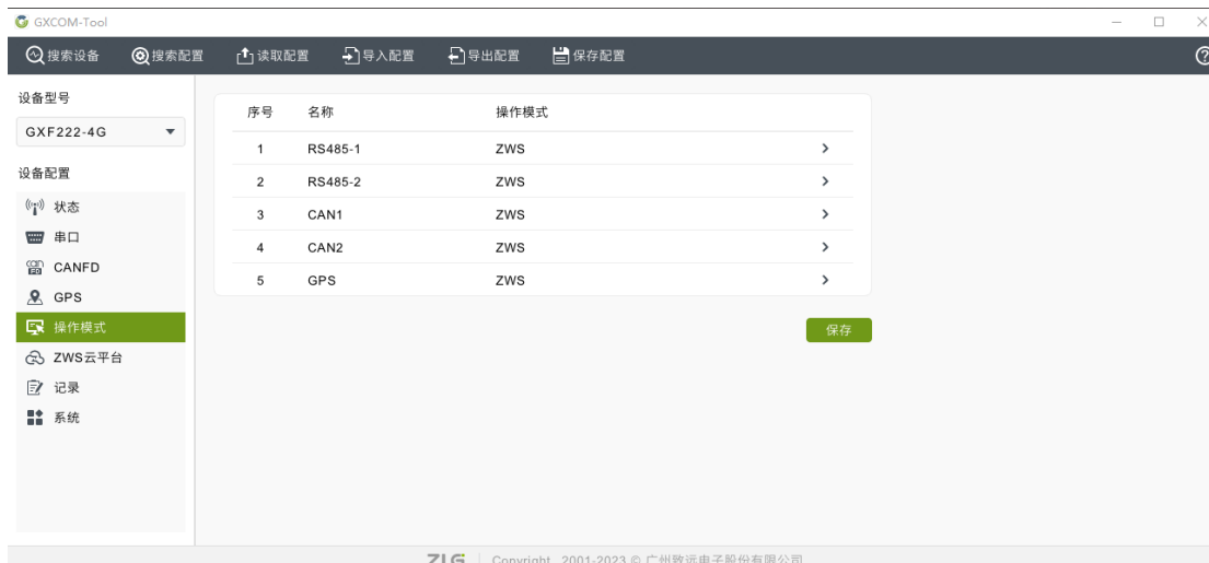
图 2.15 操作模式配置
