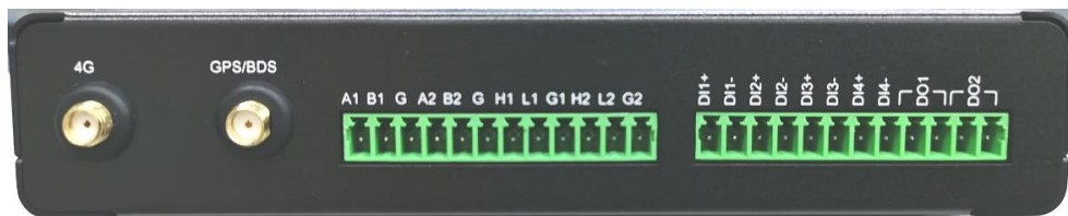
图 1.3 GXF222-4G 工业数采边缘网关底面接口图
