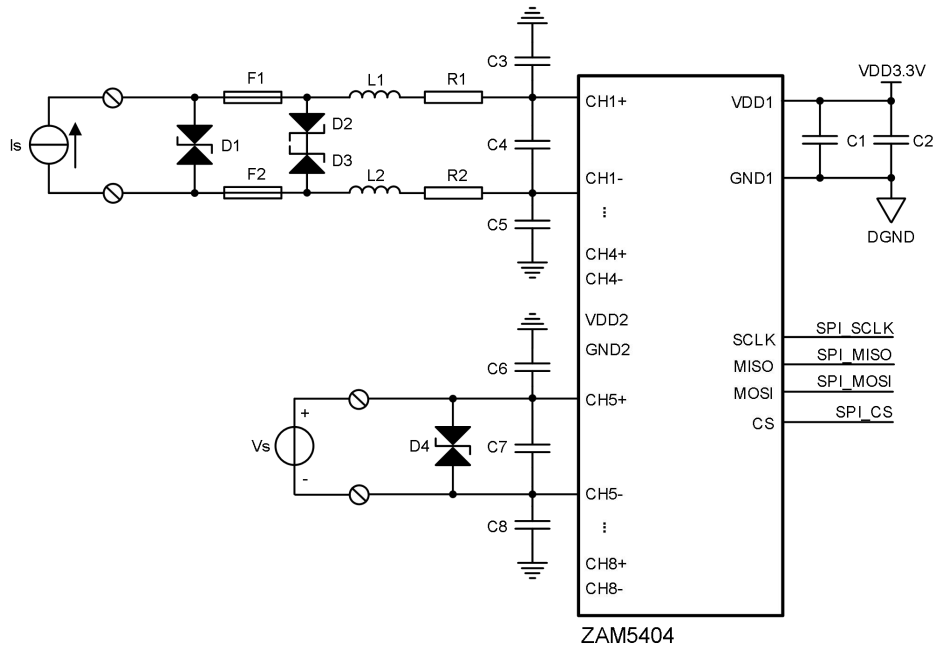
图 2.3 ZAM5404 典型应用电路
