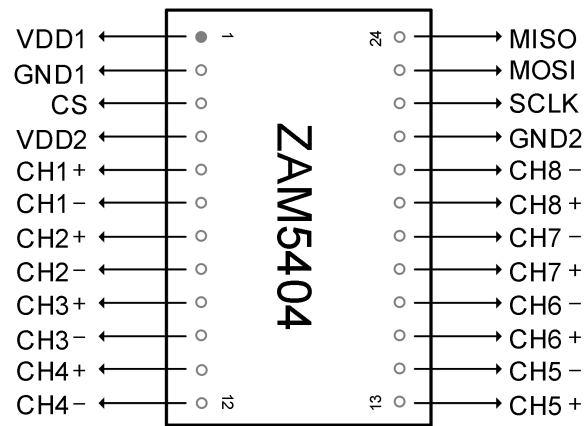
图 2.2 ZAM5404 引脚顶视图
