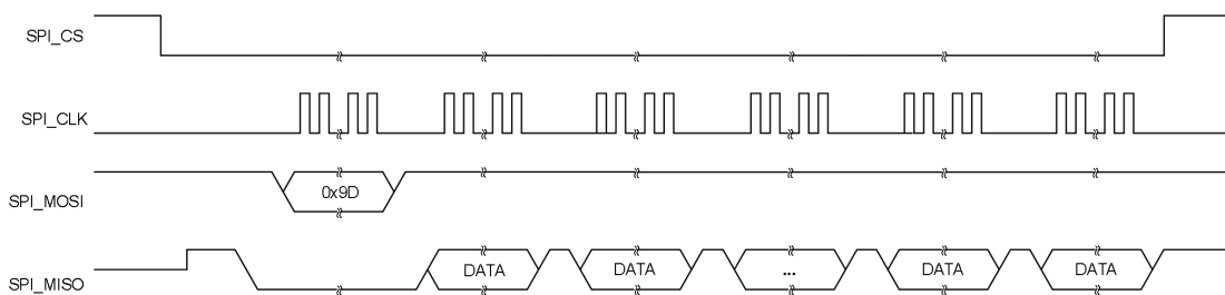
图 3.3 ZAM5404 连续模式通过中断读取 7 通道数据
