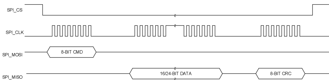
图 3.8 ZAM5404 使能 CRC 的 SPI 读处理
