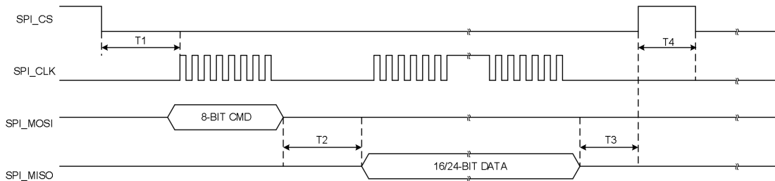
图 3.9 ZAM5404 SPI 读时序图
