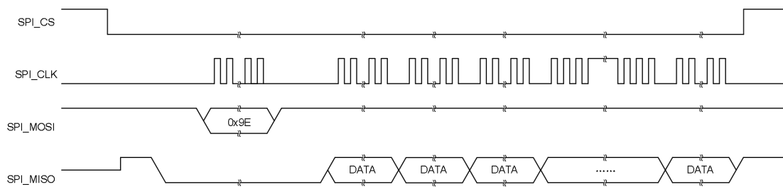
图 3.5 ZAM5404 检测 MISO 输入后开启连续转换模式
