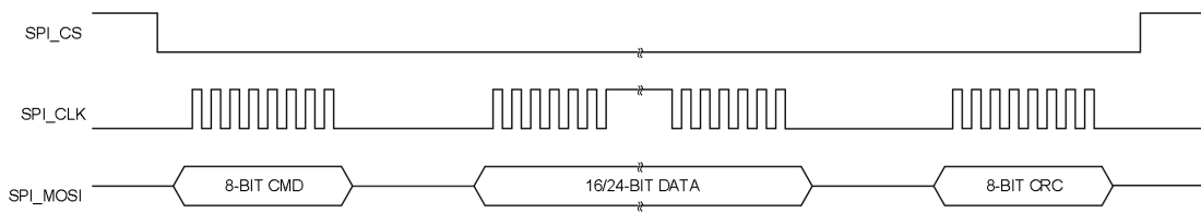
图 3.7 ZAM5404 使能 CRC 的 SPI 写处理
