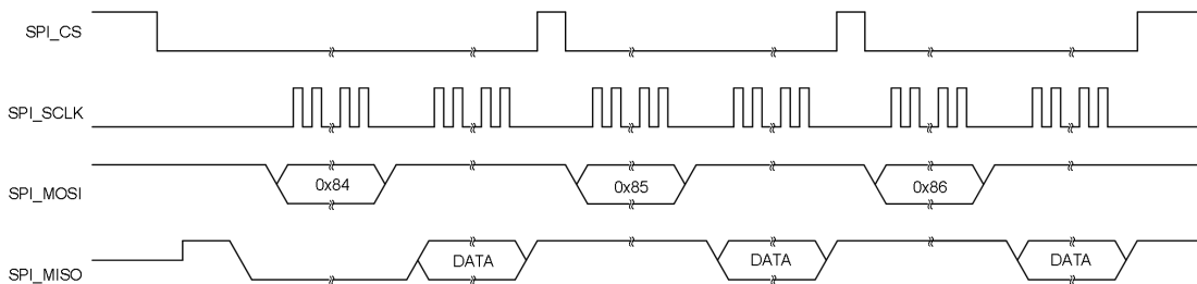
图 3.2 ZAM5404 连续模式通过中断读取所需通道数据
