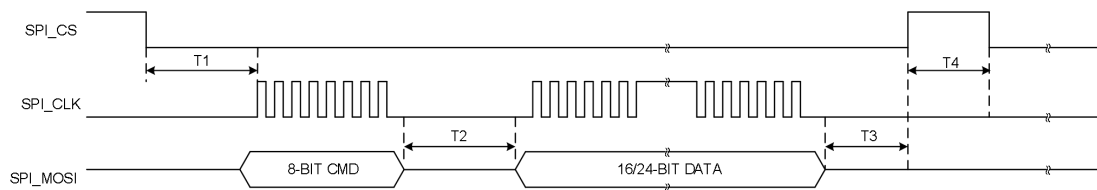
图 3.10 ZAM5404 SPI 写时序图
