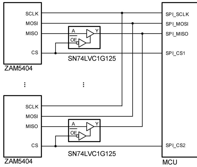
图 2.4 ZAM5404 多模块级联推荐电路
