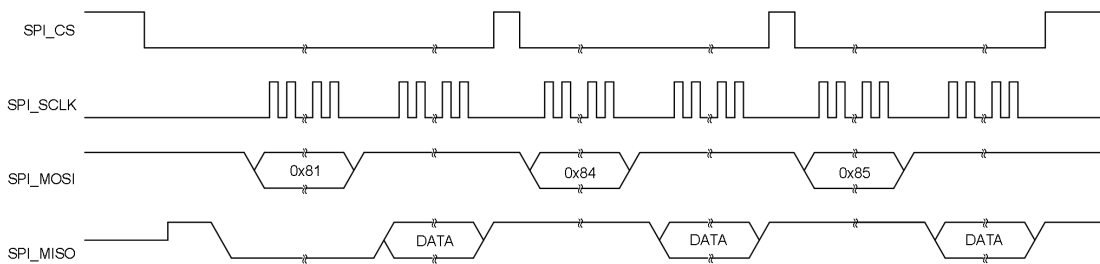
图 3.1 ZAM5404 连续转换模式通过状态寄存器读取所需通道数据
