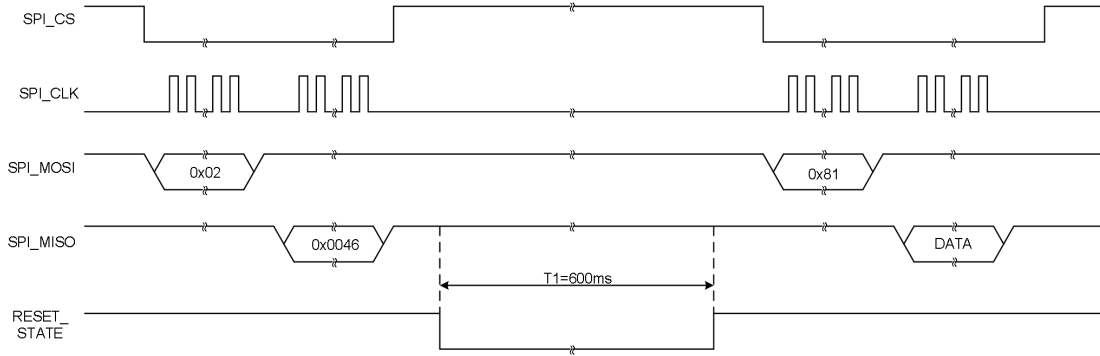
图 3.6 ZAM5404 模块复位操作及时序要求
