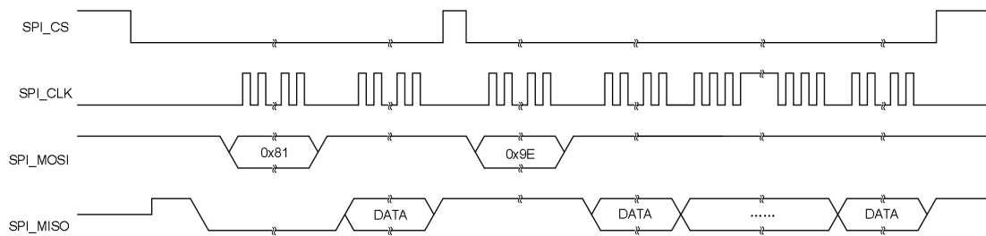
图 3.4 ZAM5404 轮询状态寄存器后开启数据缓冲模式
