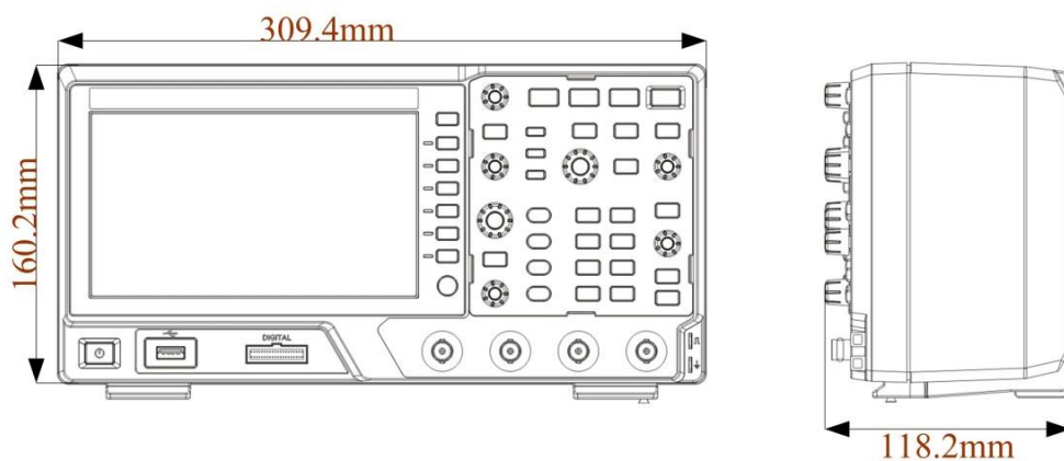
图 1 ZDS1000 外观尺寸图
