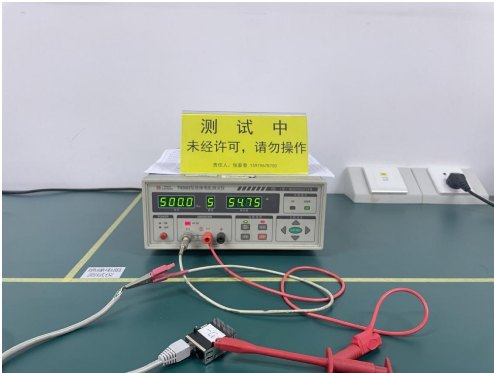
图 2 绝缘电阻试验
